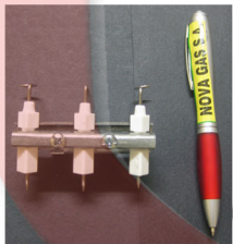
ARMADO DE BUJÍA Y SENSOR DE 07, 11, 13 Y 14 LITROS
