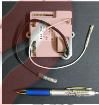
ARMADO SPARKER JUNKERS CON CABLE
