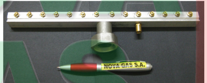
TUBO DE DISTRIBUCION GN 14 LITROS
